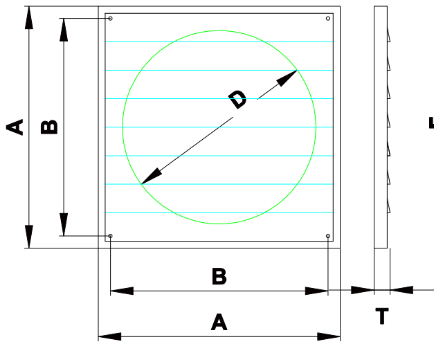
Samočinná žaluzie
