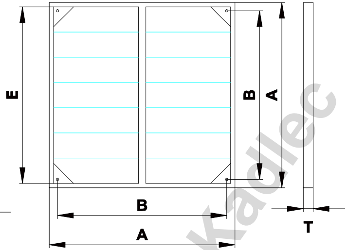
Samočinná žaluzie
